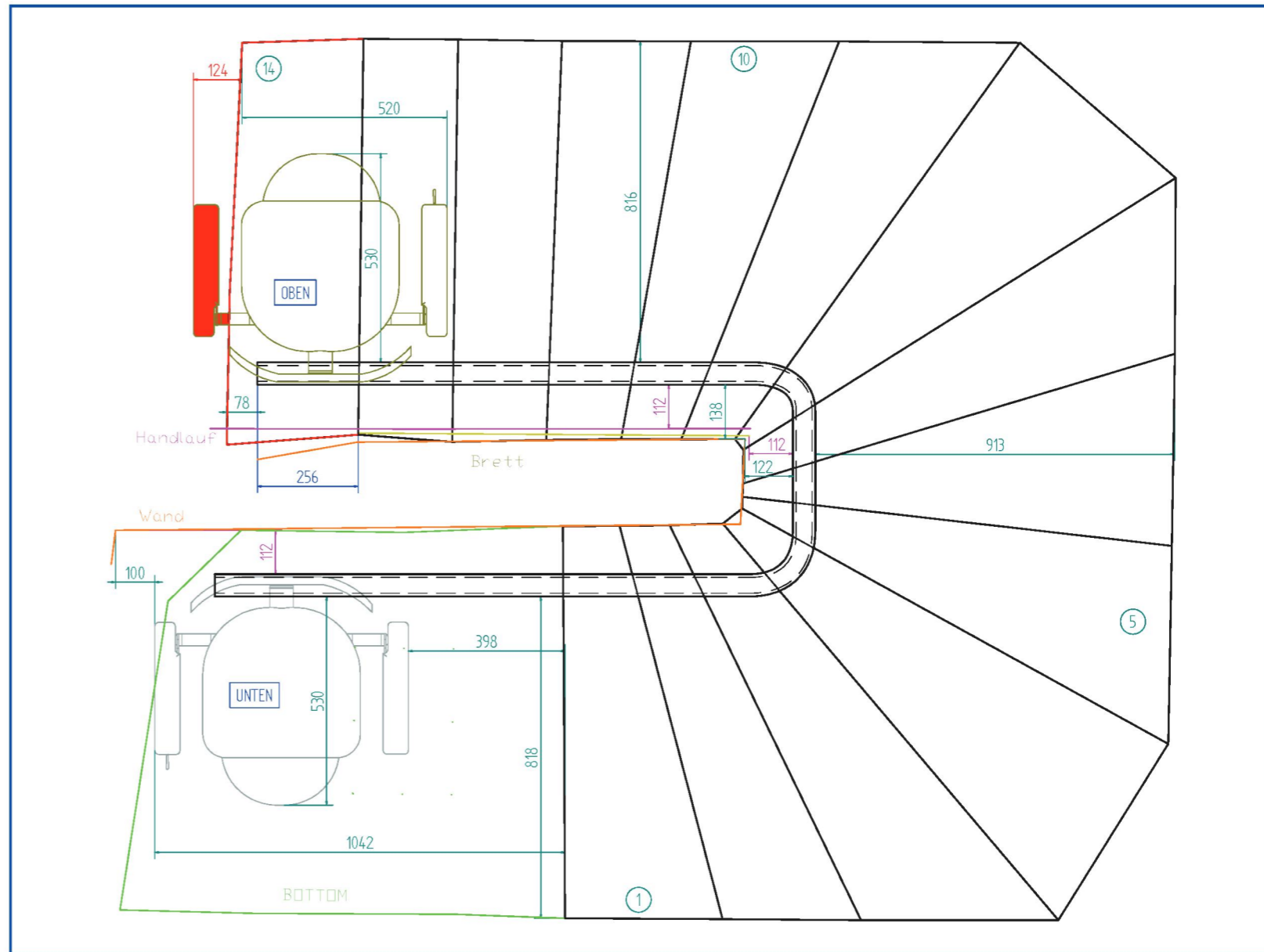
Technický list, rozmery stoličky a dráhy. Rozmery dráhy sa môžu meniť v závislosti od schodiska.
