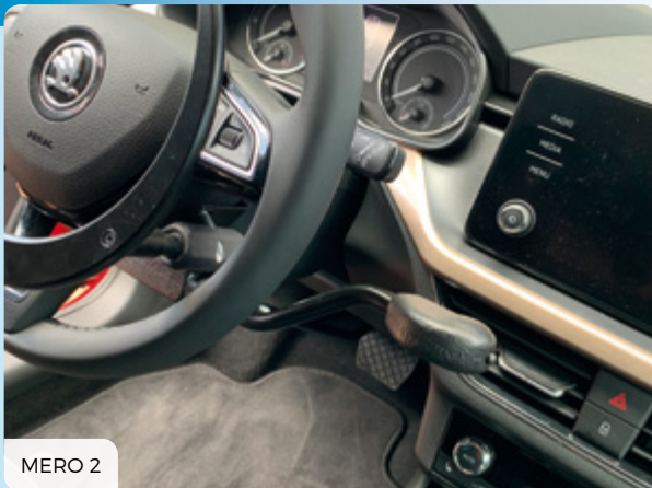
MERO 2 s prítlačným krúžkom plynu na volante
