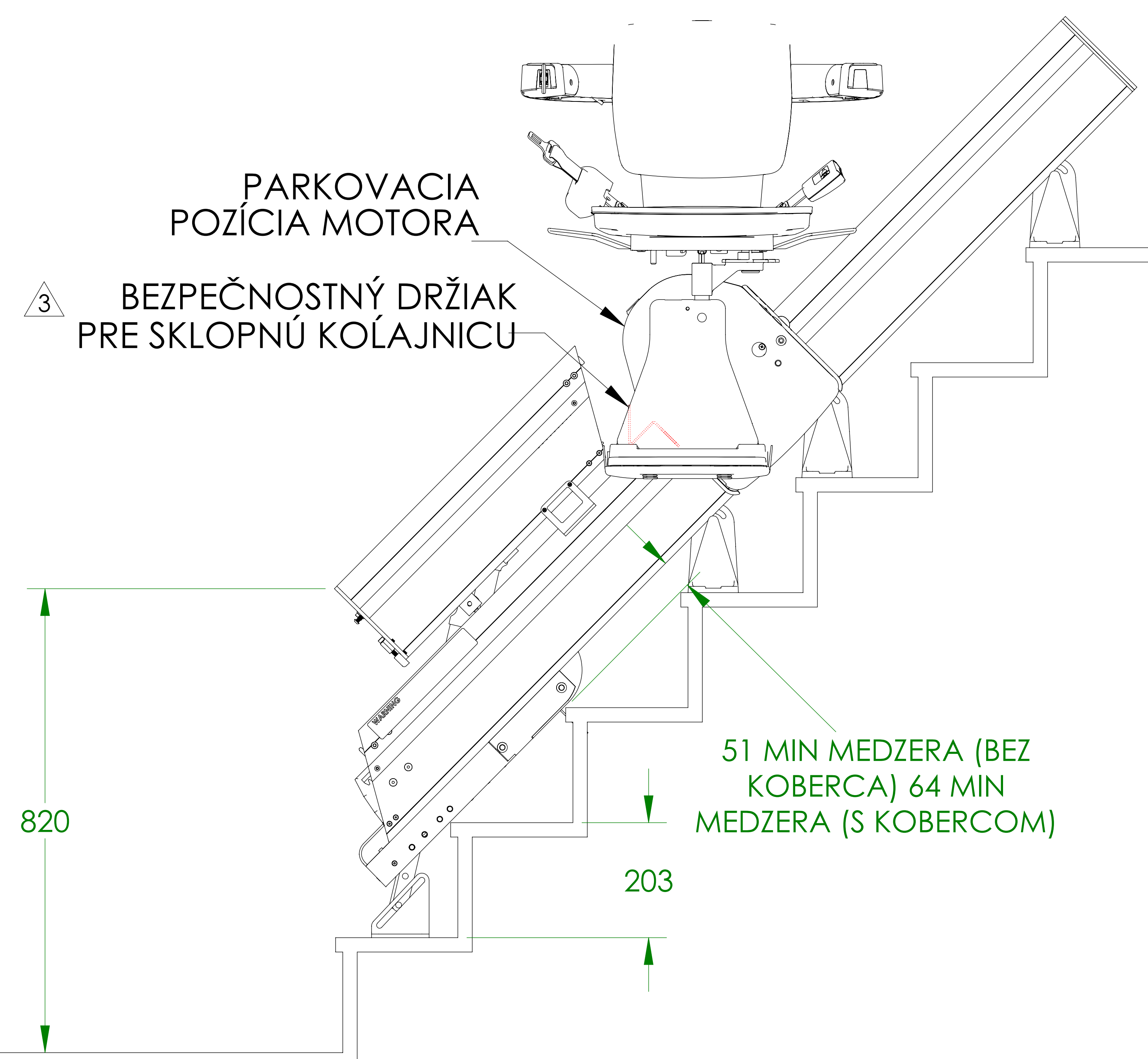
POMOCNÝ POHĽAD Z VÝŠKY NA SKLOPENÚ KOĽAJNICU
