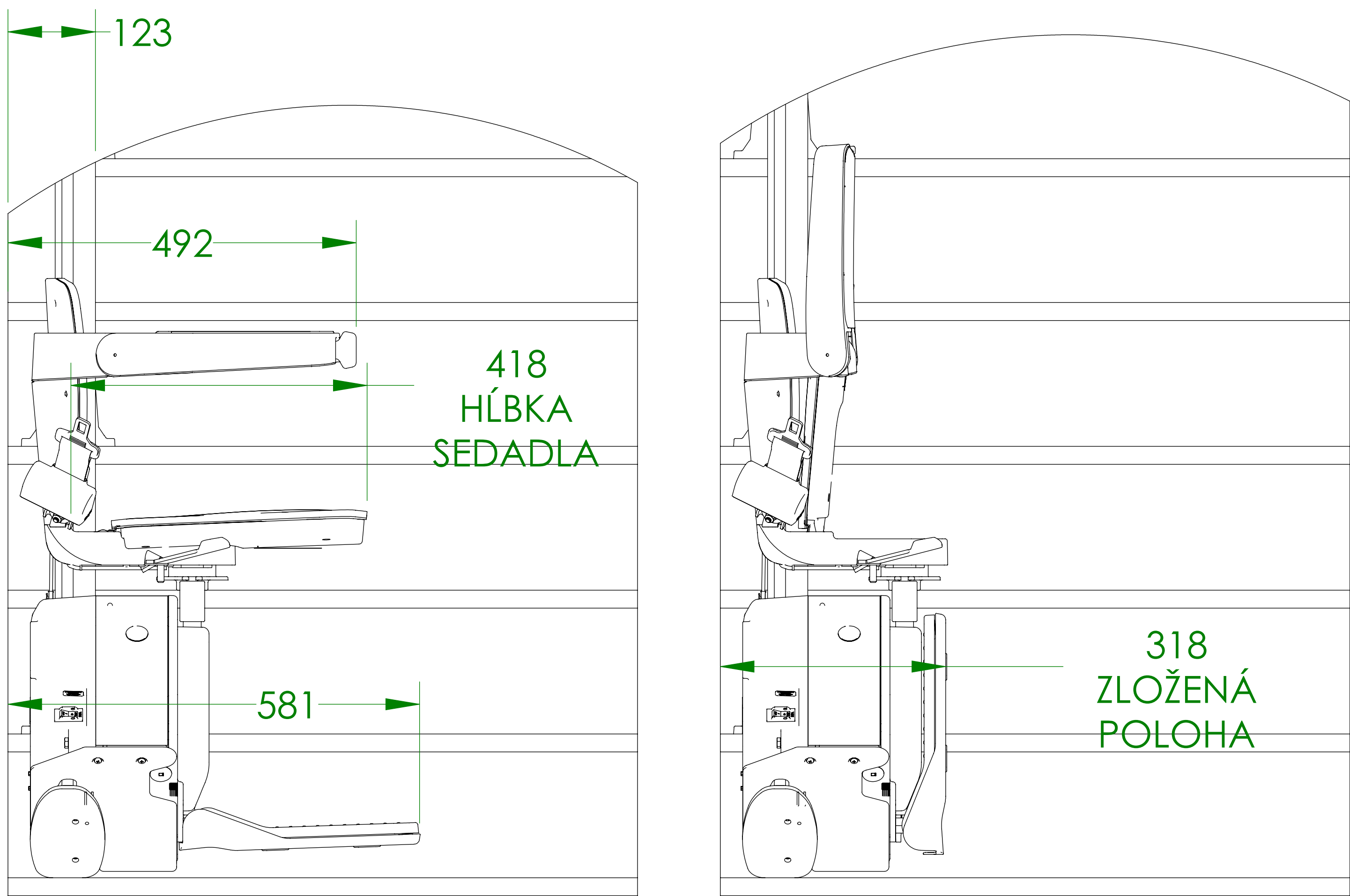
BOČNÉ POHĽADY
