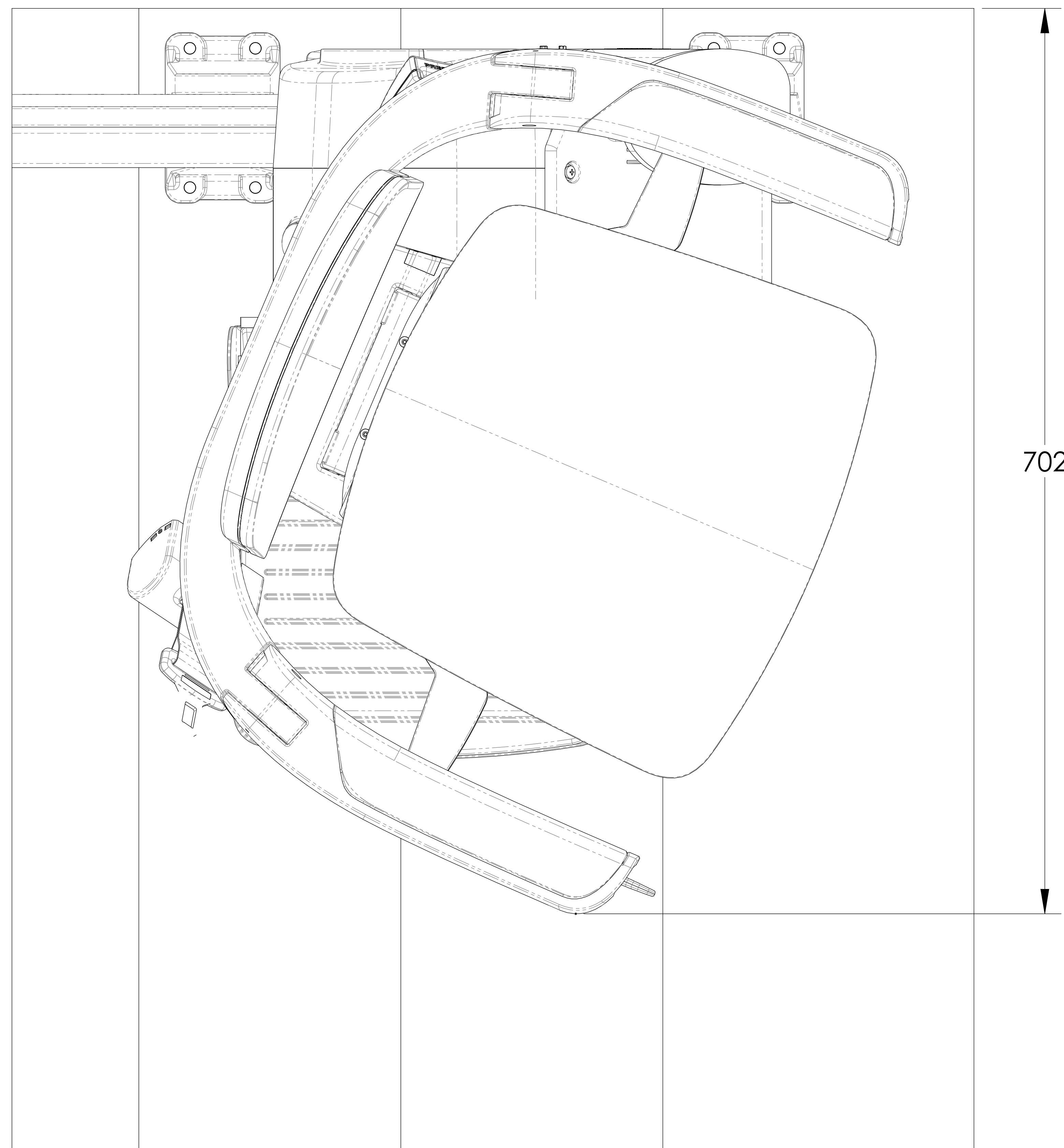
SEDADLO OTOČNÉ 67°
