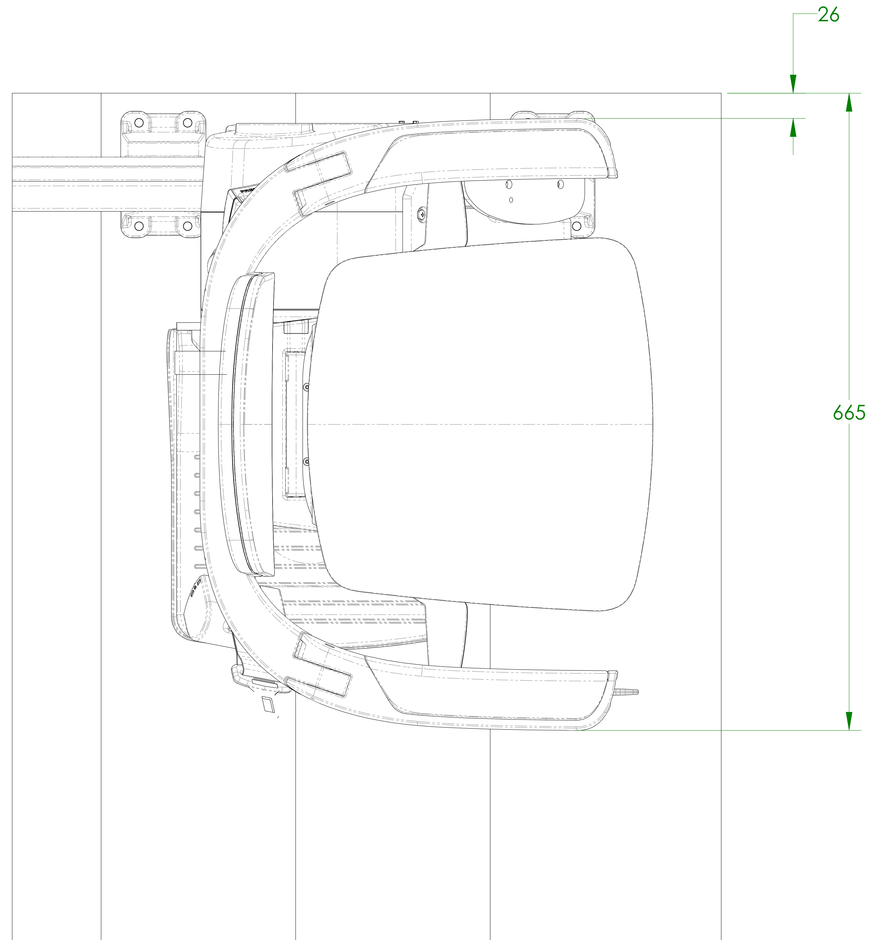
SEDADLO OTOČNÉ 90°
